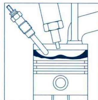
INYECCIÓN DIRECTA
