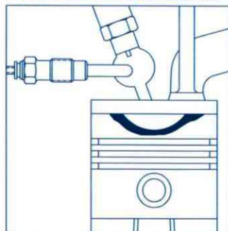
PRE COMBUSTIÓN
